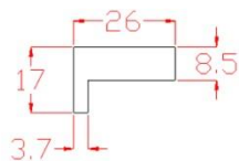
플렉시블 몰딩
